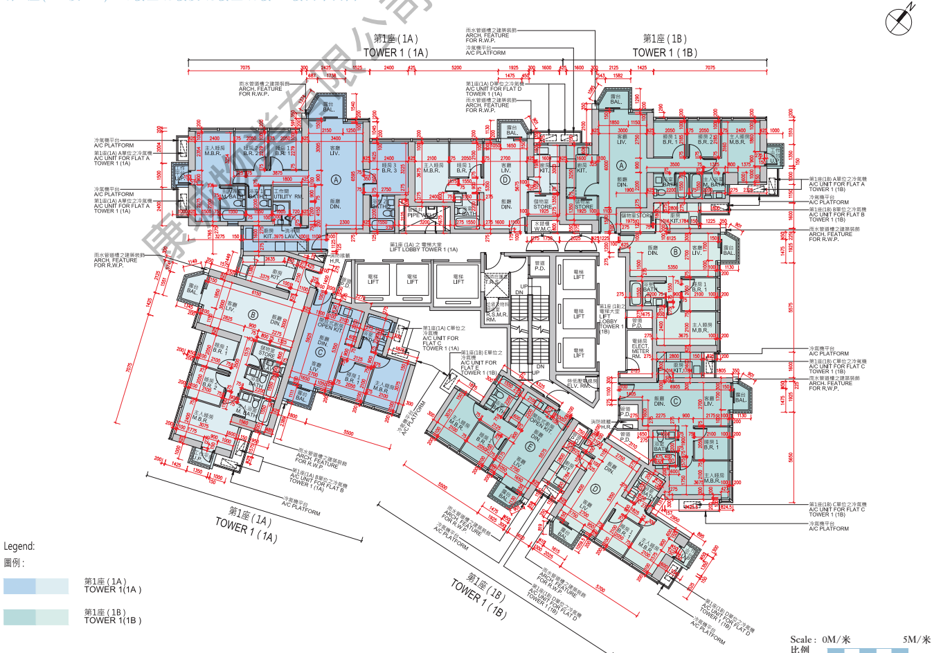
Tower 1 (1A & 1B) 17/F-23/F & 25/F-26/F Floor Plan 第1座(1A 及 1B) 17樓至23樓及25樓至26樓 樓面平面圖
